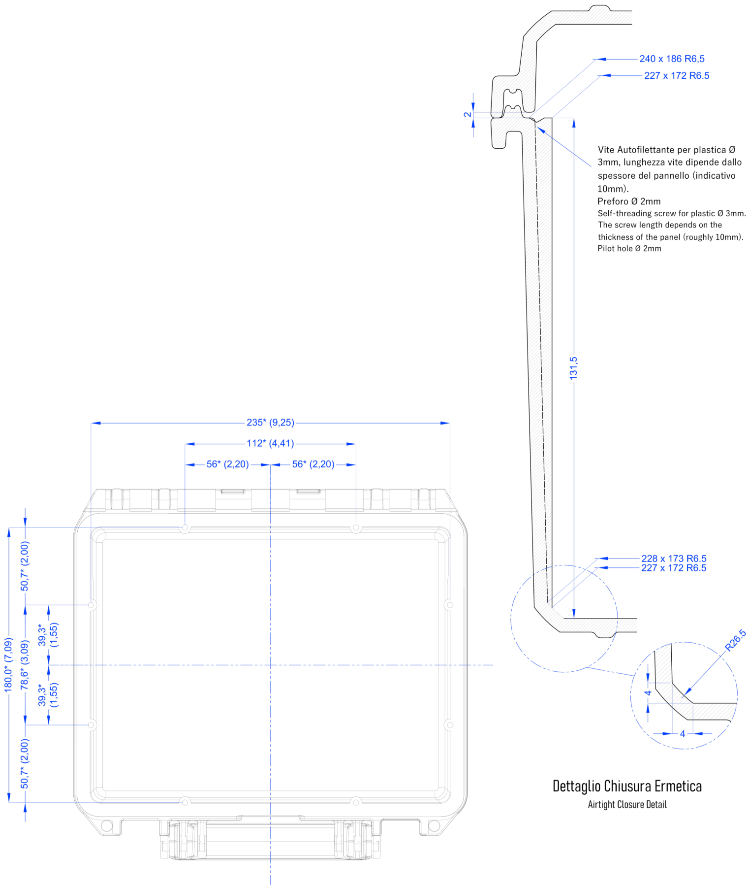
Vista Interna Fondo Bottom Inner View
