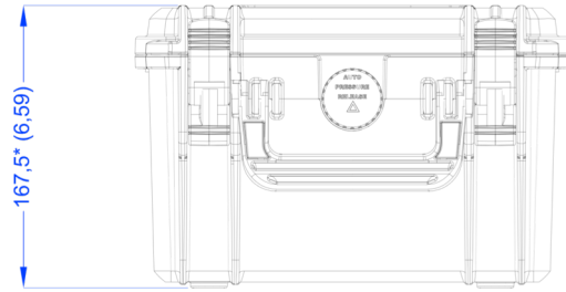
Lato Apertura Opening Side
